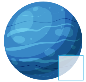
Нептун
