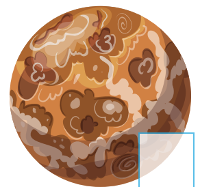
Венера
