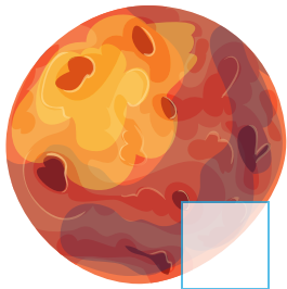
Марс
