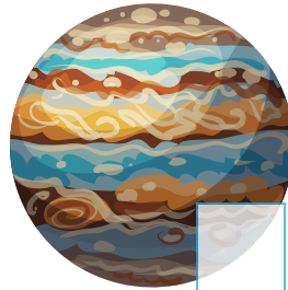
Юпітер
