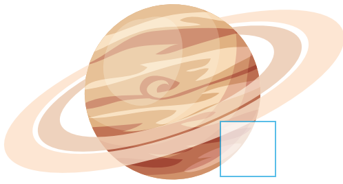
Сатурн
